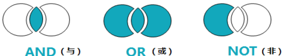
图 2-34 逻辑运算符
